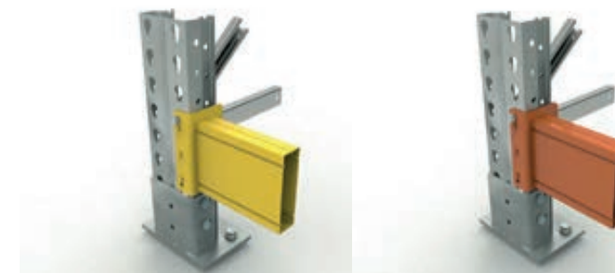
► Galvanizado por inmersión en Caliente + Pintura electroestática en polvo Hot dip galvanized + Electrostatic powder coating
